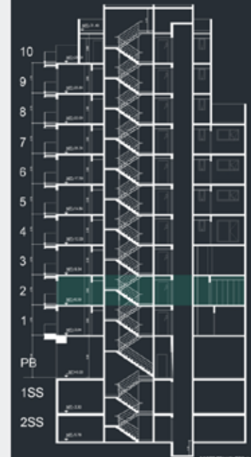
2° PISO
