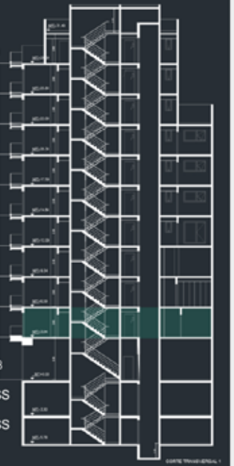
1° PISO
