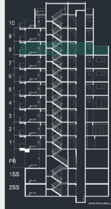
8° PISO
